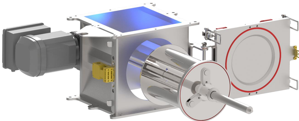
RO-3-60-SR Standard mit gezogener Magneinheit mittels Kombigriff
